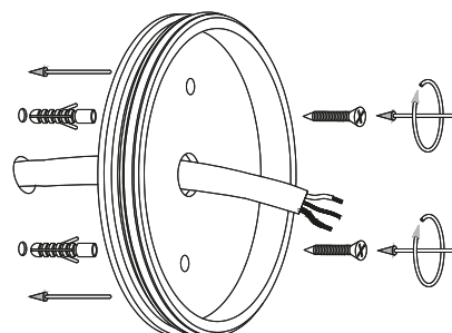
3 - Instalar la placa base
